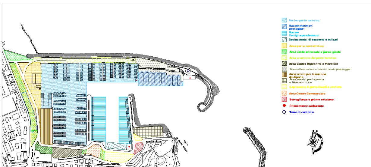
5.2. Piano Regolatore Portuale: Planimetria generale
