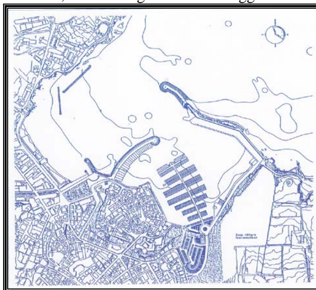
1.4. Progetto preliminare generale del porto turistico
