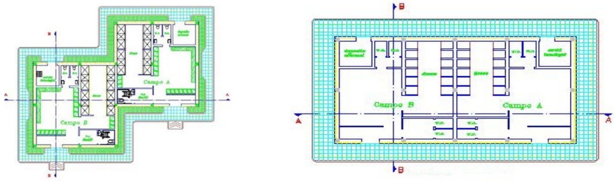
13.2. Piante e prospetto spogliatoi basket e calcetto
